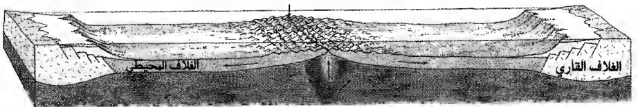
مرحلة تكون المحيط حافة وسط المحيط أخدود
